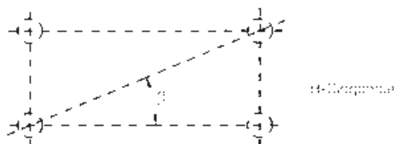
Bild 3. Statisches System Horizontal-diagonalanschluß
