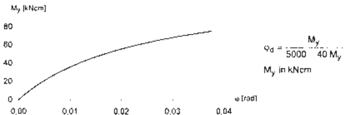
Bild 3: Minimale Drehfedersteifigkeit
