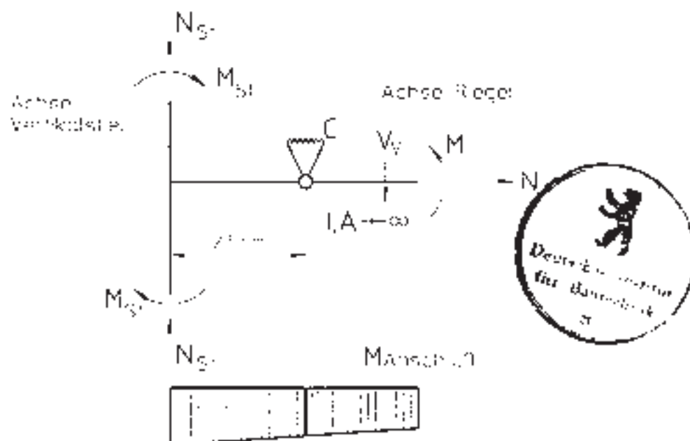
Bild 1. Statisches System Riegelanschluß
