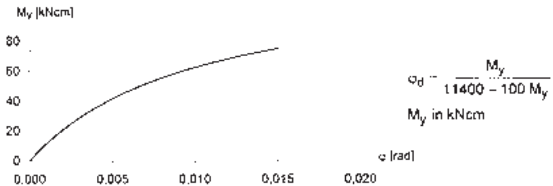
Bild 1: Mittlere Drehfedersteifigkeit
