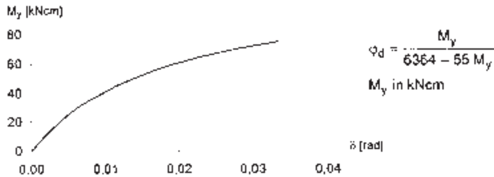
Bild 4: Reduzierte Drehfedersteifigkeit
